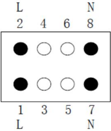
图 4 FC3280W1 连接的电能表载波耦合接口示意图
