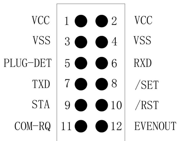
图 3 与 FC3280W1 连接的电能表弱电接口示意图
