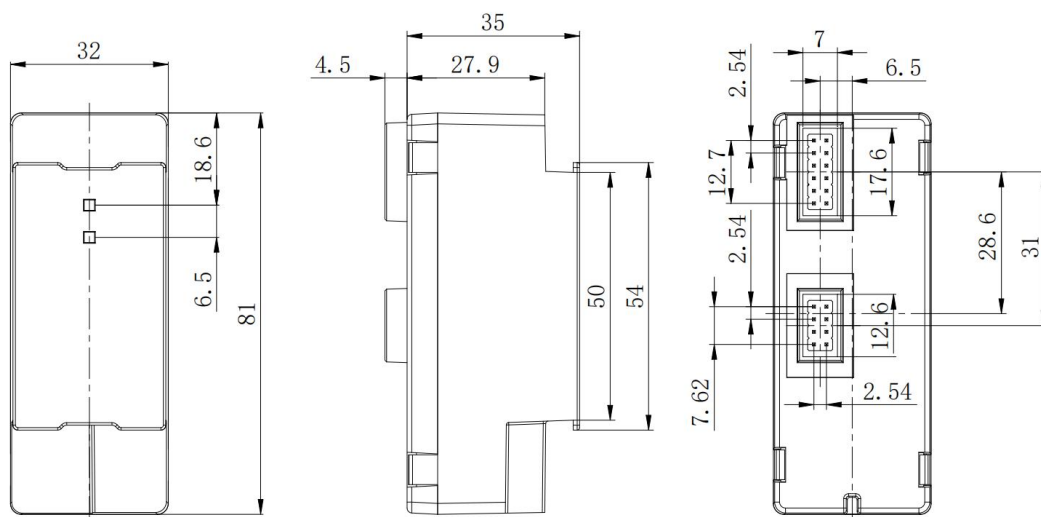
图 1 产品尺寸图
