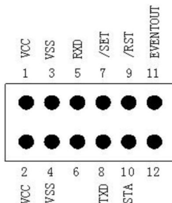
图 3 与 FC3280B1 连接的电能表弱电接口示意图
