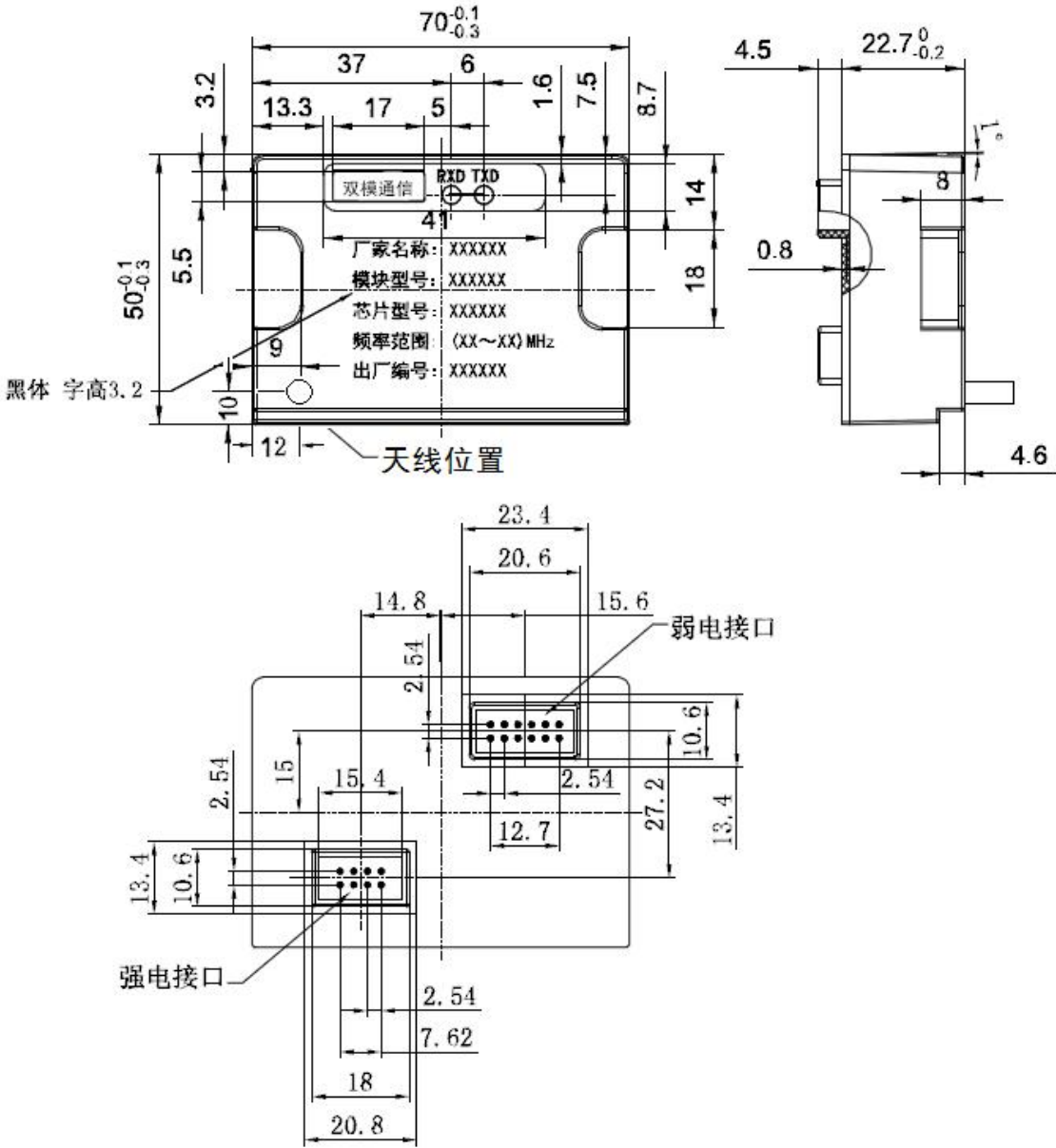
图 1 产品尺寸图
