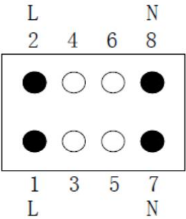
图 4 FC3280B1 连接的电能表载波耦合接口示意图
