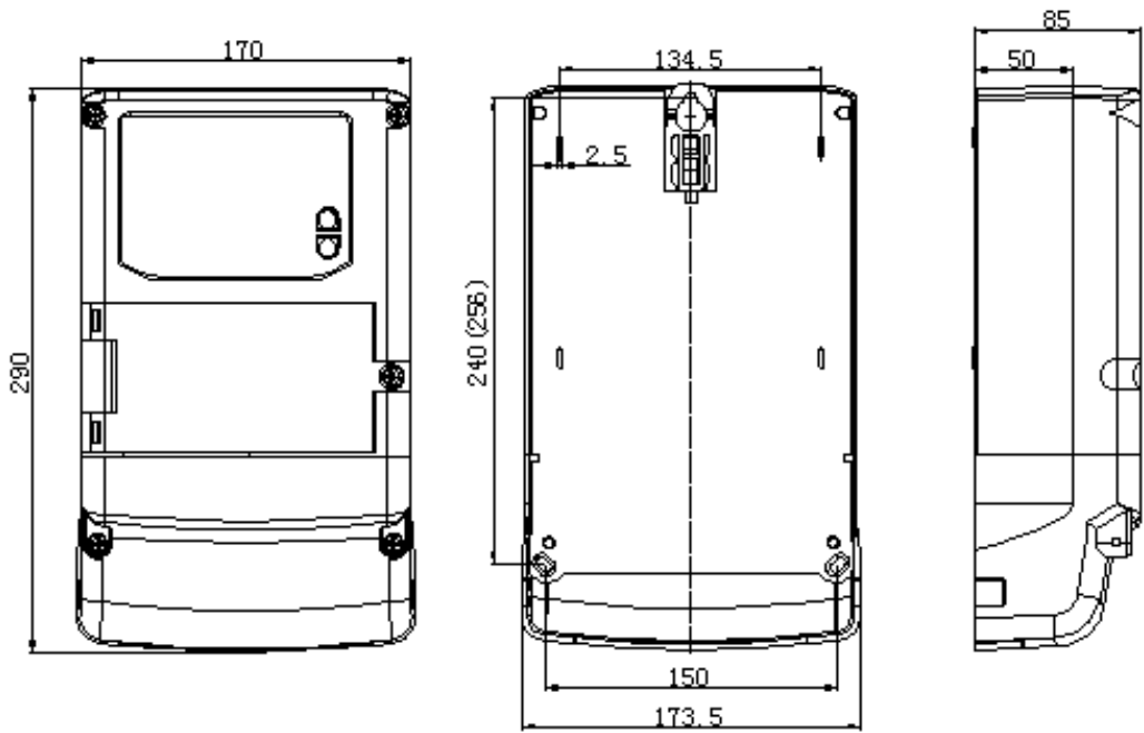
外形图
