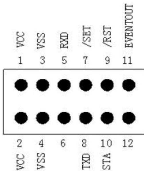
图 3 与 FC3280B3 连接的电能表弱电接口示意图
