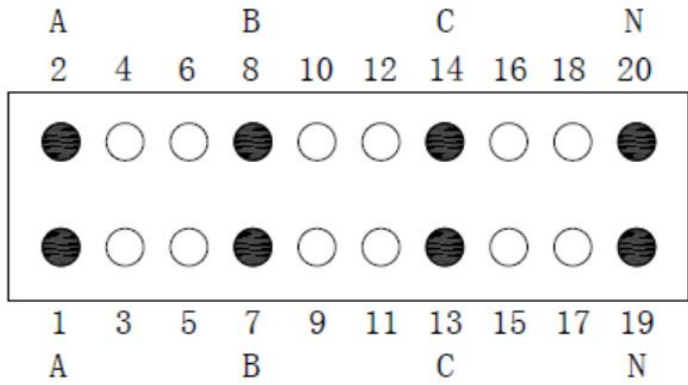
图 4 与 FC3280B3 模块连接电能表载波耦合接口示意图
