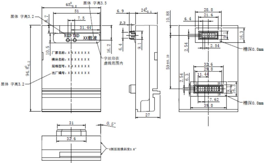
图 1 产品尺寸图
